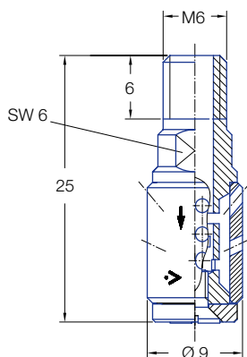
Außengewinde
