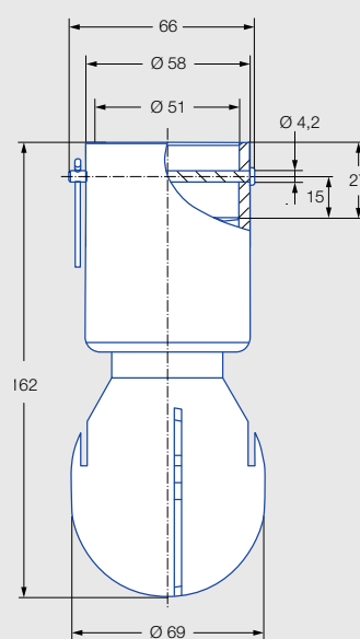
Abmessungen der 2" -Steckverbindungen gemäß ASME-BPE (OD-Tube)
