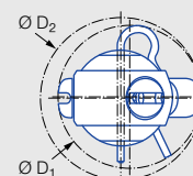
Einführdurchmesser D_1 und Störkreisdurchmesser D_2 der Steckverbindung
