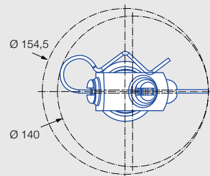
Einführdurchmesser und Störkreisdurchmesser der Steckverbindung
