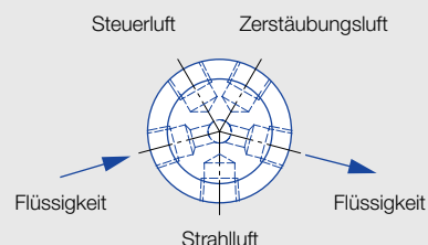
Ausführung mit 5 Anschlüssen
