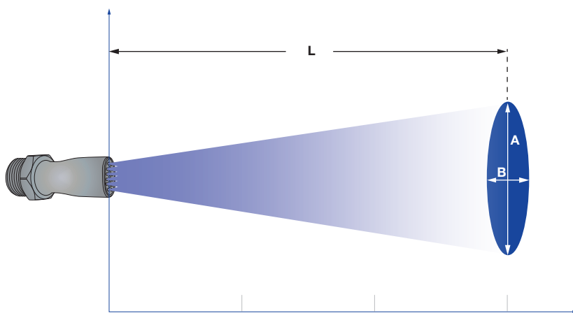
Strahlausbreitung der Baureihe 600.386.01.AE
