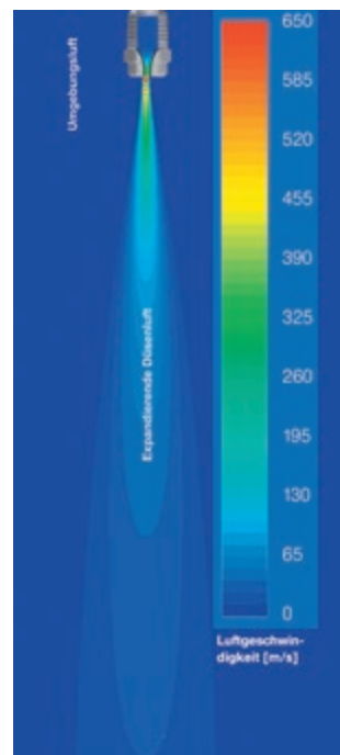
Abbildung 4: Darstellung des Geschwindigkeitsverlaufes von ausströmender Luft
