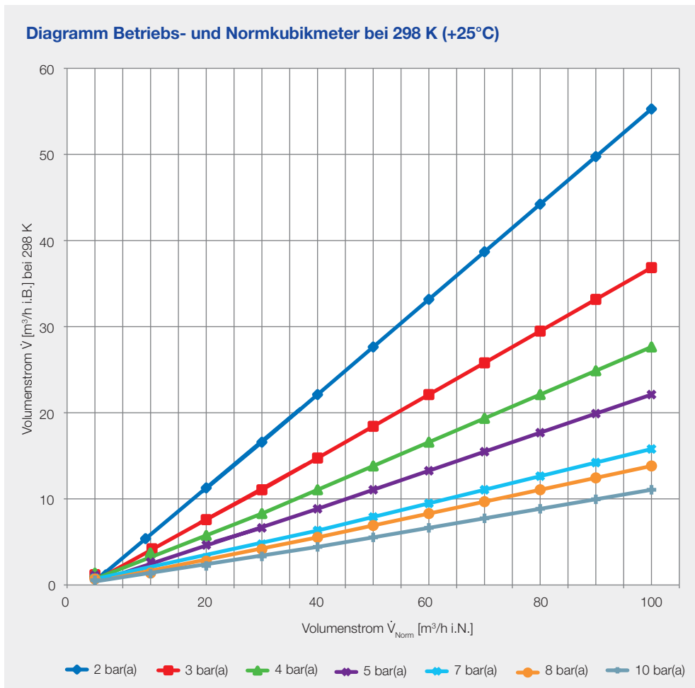
Abbildung 1: Zusammenhang zwischen Norm- und Betriebsvolumenstrom
