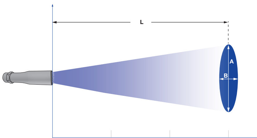
Strahlausbreitung der Baureihe 600.382.35.AE
