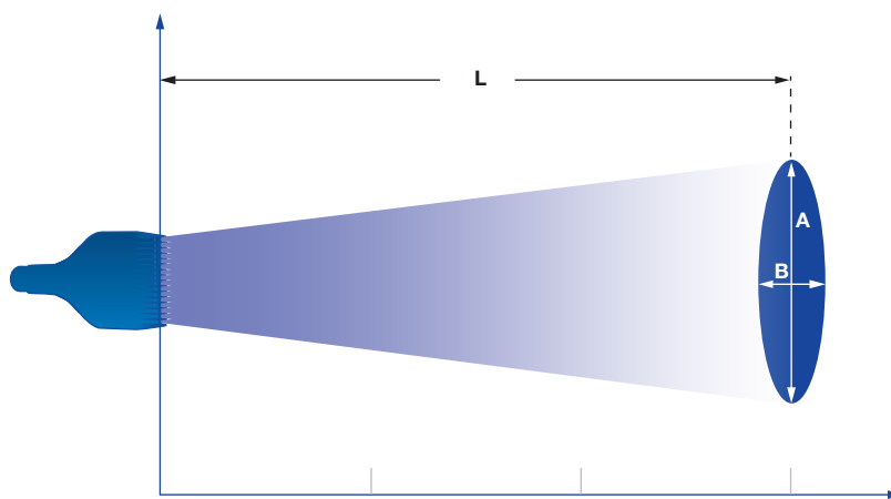
Strahlausbreitung der Baureihe 600.332
