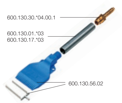
600.130.56.01 mit Zubehör *01 = 1.0711 / 17 = AISI 316Ti / 30 = Messing
