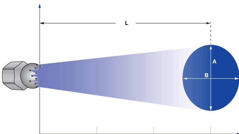
Strahlausbreitung der Baureihen 540 / 541
