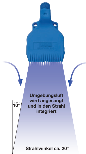
Abbildung 2: Strahlaufweitung einer Druckluftdüse
