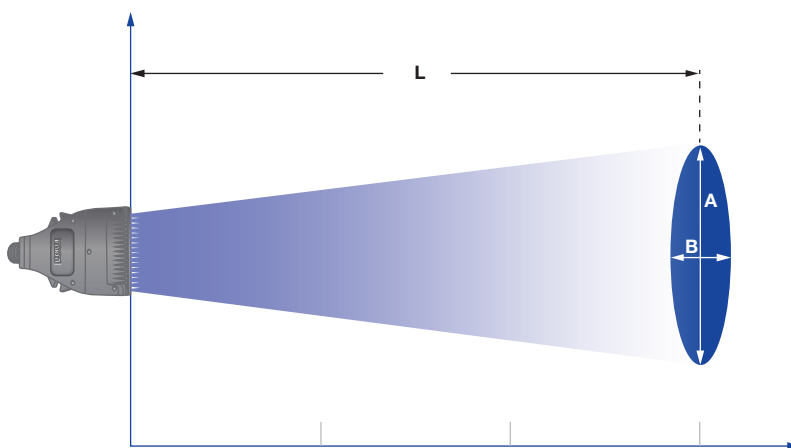
Strahlausbreitung der Baureihe 600.283
